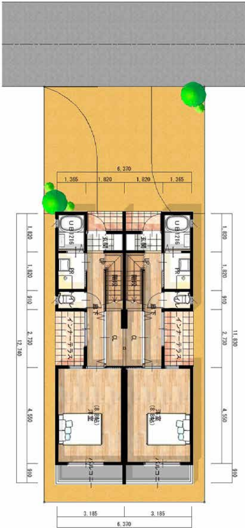
1階 平面図
